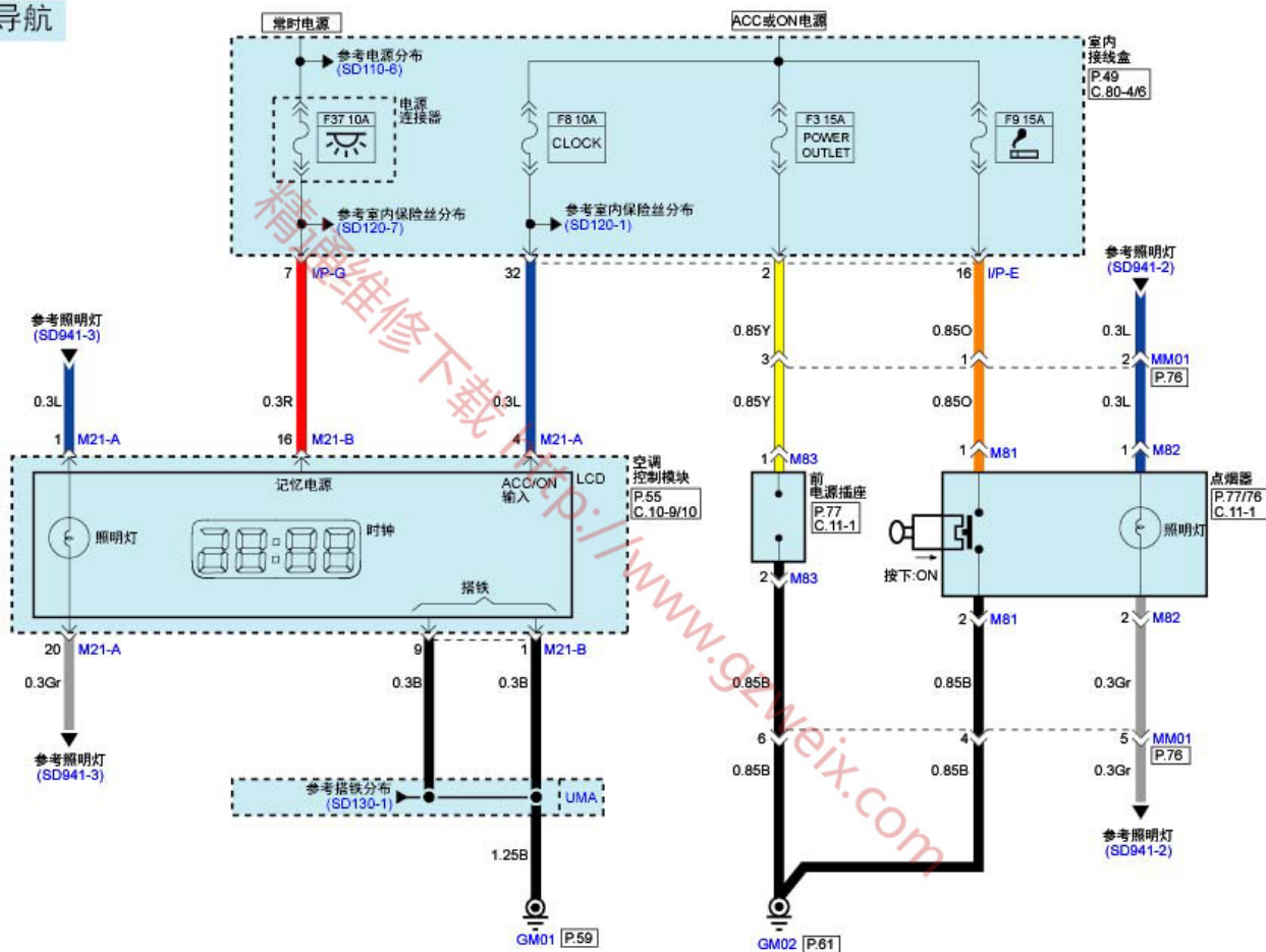
时钟&amp;点烟器(电源插座)系统(1)
